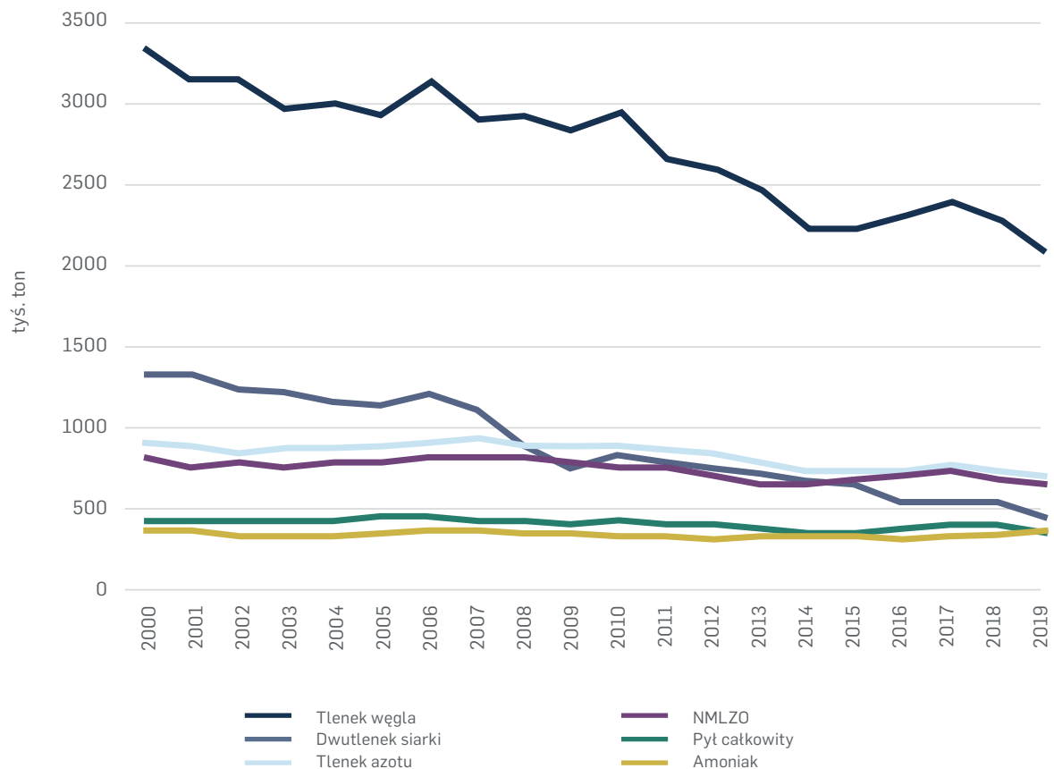
Wykres 8. Całkowita emisja głównych zanieczyszczeń powietrza
